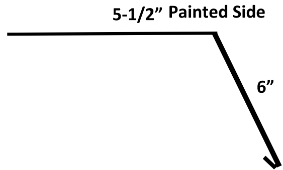
Fascia 10'L
